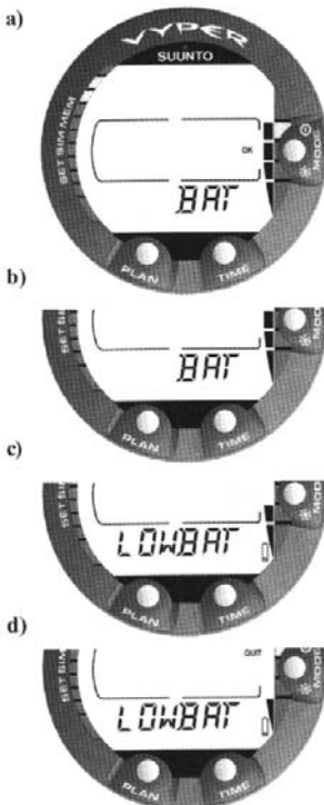
איור 3.2 הדלקה II. חיווי מצב הסוללה.
