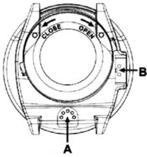
איור 2.3 חיישן העומק A, מגע מים/מחבר העברת מידע B.
